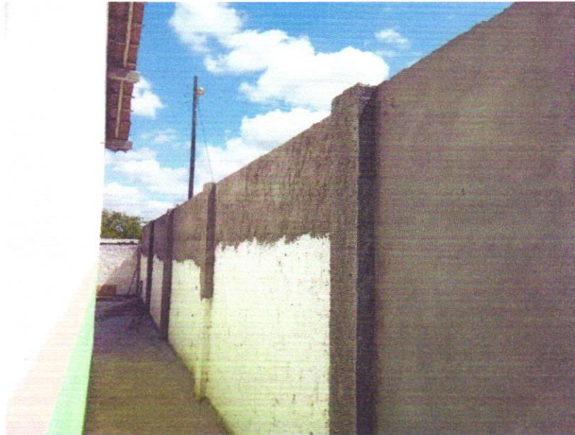
FOTO 03 - CHAPISCO APLICADO EM ALVENARIA (COM PRESENÇA DE VÃOS) E ESTRUTURAS DE CONCRETO DE FACHADA, COM COLHER DE PEDREIRO. ARGAMASSA TRAÇO 1:3 COM PREPARO EM BETONEIRA 400L. AF_10/2022
